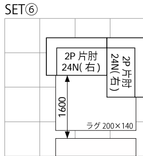
W2465 D1510
